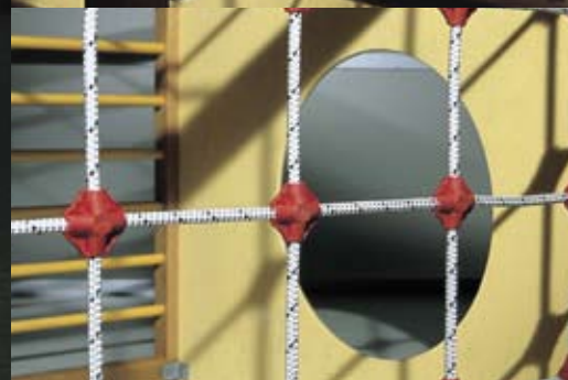
giunti in nylon per tenere le corde in tensione
